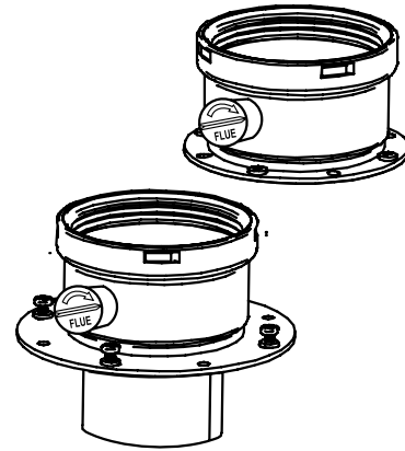
Adaptateurs pour systèmes séparés
