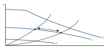
Fig. 28 Trois réglages courbe constante/vitesse constante
