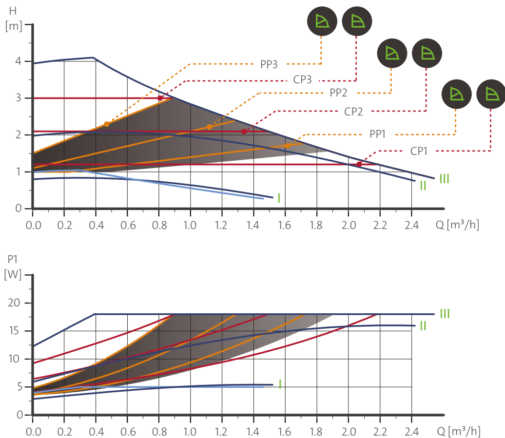
Fig. 37 ALPHA2 et ALPHA3, XX-40
