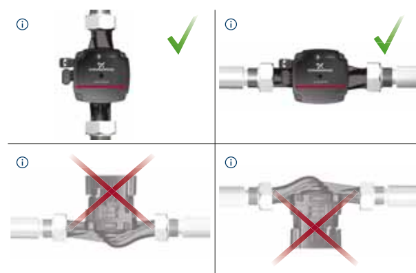
Fig. 7 Position du coffret de commande de l'ALPHA SOLAR
