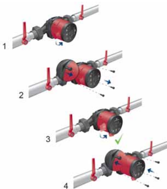
Fig. 5 Modification de la position du coffret de commande
