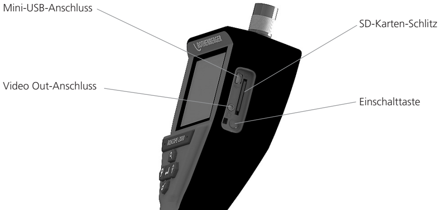
Bild Nr. 14 – USB-Verbindung für Übertragungen
