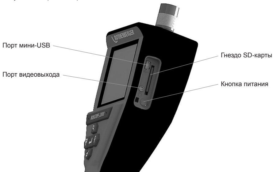
Рисунок 11 – Входы/выходы прибора
