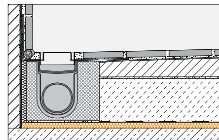
Schlüter®-KERDI-LINE-SR (Exemple de montage KERDI-LINE-H 40, configuration B, voir « Base de planification Schlüter®-KERDI-LINE-SR »)
