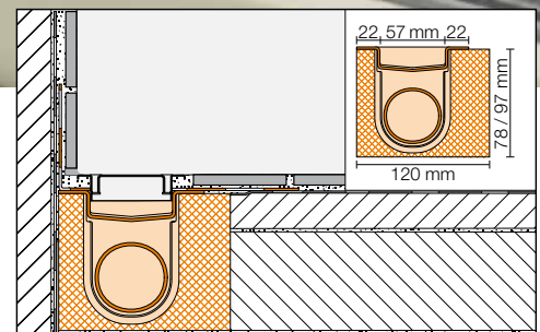
Schlüter®-KERDI-LINE-H (ci-dessus avec cadre standard)
