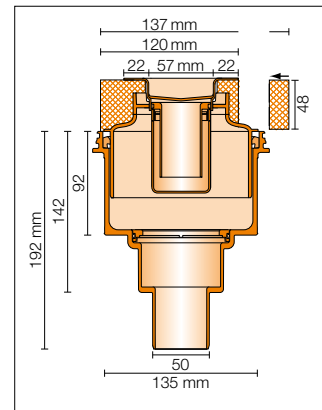
Coupe transversale
