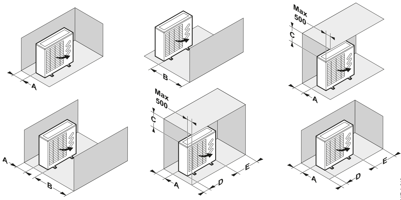
Fig.21 Distances d'implantation
